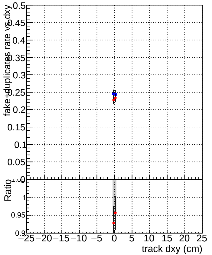
DQM_CKF_XiMinusNOPU_base DQM_CKF_XiMinusNOPU_retrainOldFiles125_v2_prelimWPM_epoch4
