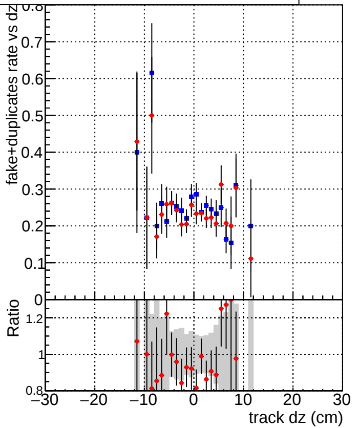
DQM_CKF_XiMinusNOPU_base DQM_CKF_XiMinusNOPU_retrainOldFiles125_v2_prelimWPM_epoch4
