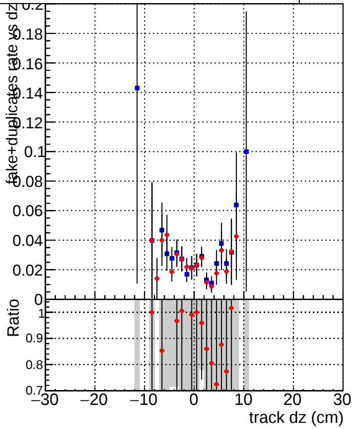
Legend: ■ DQM_CKF_XiMinusNOPU_base ● DQM_CKF_XiMinusNOPU_retrainOldFiles125_v2_prelimWPM_epoch4
