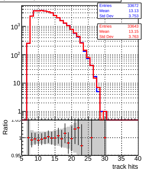
mean hits — DQM_CKF_XiMinusNOPU_base — DQM_CKF_XiMinusNOPU_retrainOldFiles125_v2_prelimWPM_epoch4
