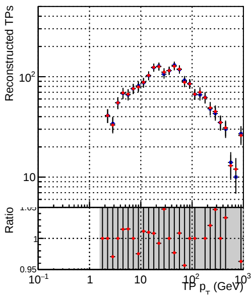
—●— DQM_CKF_XiMinusNOPU_base —●— DQM_CKF_XiMinusNOPU_retrainOldFiles125_v2_prelimWPM_epoch4
