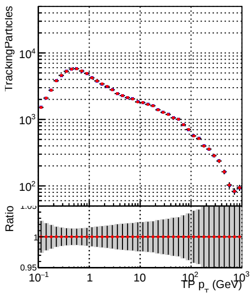
—●— DQM_CKF_XiMinusNOPU_base —●— DQM_CKF_XiMinusNOPU_retrainOldFiles125_v2_prelimWPM_epoch4
