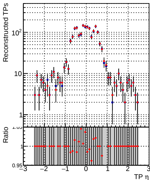
—●— DQM_CKF_XiMinusNOPU_base —●— DQM_CKF_XiMinusNOPU_retrainOldFiles125_v2_prelimWPM_epoch4
