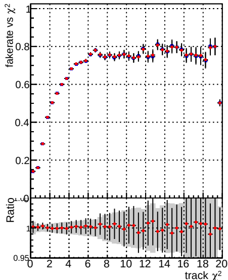
Fake rate vs. \chi^2 —•— DQM CKF XiMinusNOPU_base —•— DQM CKF XiMinusNOPU_retrainOldFiles125_v2_prelimWPM_epoch4
