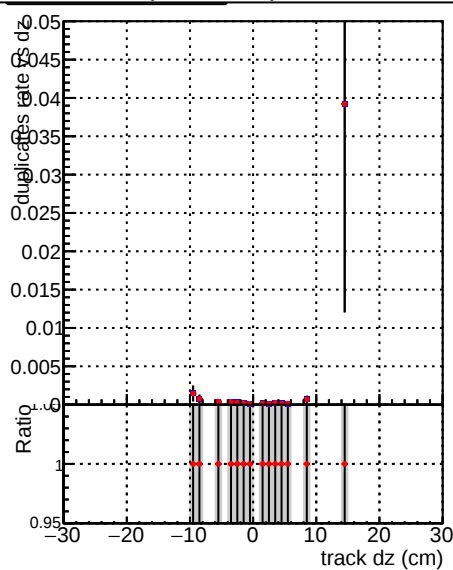
—•— DQM_CKF_XiMinusNOPU_base —•— DQM_CKF_XiMinusNOPU_retrainOldFiles125_v2_prelimWPM_epoch4
