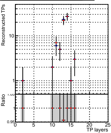
■ DQM_CKF_XiMinusNOPU_base ■ DQM_CKF_XiMinusNOPU_retrainOldFiles125_v2_prelimWPM_epoch4
