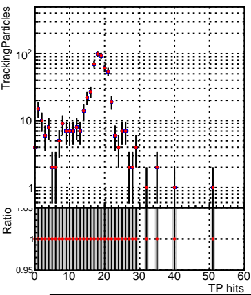
■ DQM_CKF_XiMinusNOPU_base ■ DQM_CKF_XiMinusNOPU_retrainOldFiles125_v2_prelimWPM_epoch4
