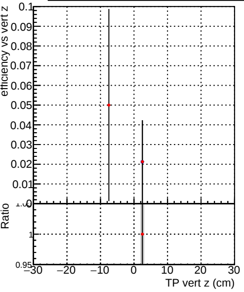
Efficiency vs vert z Legend: DQM_CKF_XiMinusNOPU_base DQM_CKF_XiMinusNOPU_retrainOldFiles125_v2_prelimWPM_epoch4
