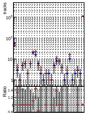
— DQM_CKF_XiMinusNOPU_base — DQM_CKF_XiMinusNOPU_retrainOldFiles125_v2_prelimWPM_epoch4
