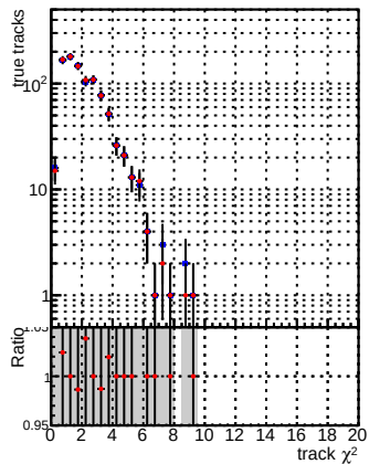
— DQM_CKF_XiMinusNOPU_base — DQM_CKF_XiMinusNOPU_retrainOldFiles125_v2_prelimWPM_epoch4
