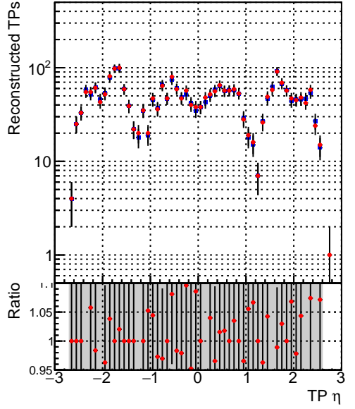
■ DQM_CKF_XiMinusNOPU_base ● DQM_CKF_XiMinusNOPU_retrainOldFiles125_v2_prelimWPM_epoch4
