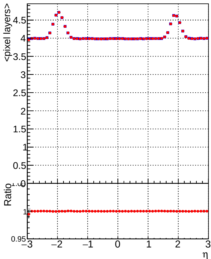
—■— DQM_CKF_XiMinusNOPU_base —●— DQM_CKF_XiMinusNOPU_retrainOldFiles125_v2_prelimWPM_epoch4
