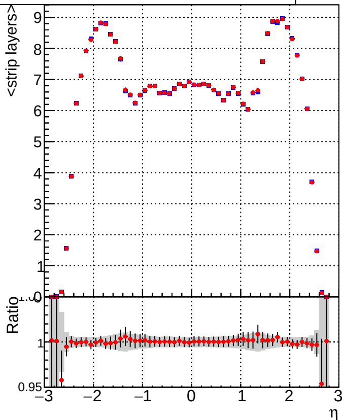
—■— DQM_CKF_XiMinusNOPU_base —●— DQM_CKF_XiMinusNOPU_retrainOldFiles125_v2_prelimWPM_epoch4
