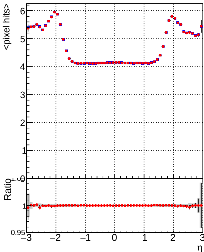
—■— DQM_CKF_XiMinusNOPU_base —●— DQM_CKF_XiMinusNOPU_retrainOldFiles125_v2_prelimWPM_epoch4
