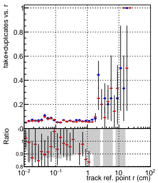
■ DQM_CKF_XiMinusNOPU_base ● DQM_CKF_XiMinusNOPU_retrainOldFiles125_v2_prelimWPM_epoch4
