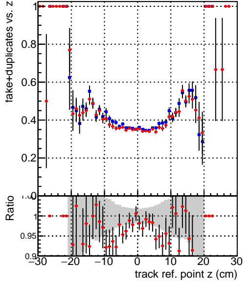
■ DQM_CKF_XiMinusNOPU_base ● DQM_CKF_XiMinusNOPU_retrainOldFiles125_v2_prelimWPM_epoch4
