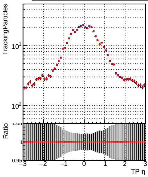
—●— DQM_CKF_XiMinusNOPU_base —●— DQM_CKF_XiMinusNOPU_retrainOldFiles125_v2_prelimWPM_epoch4
