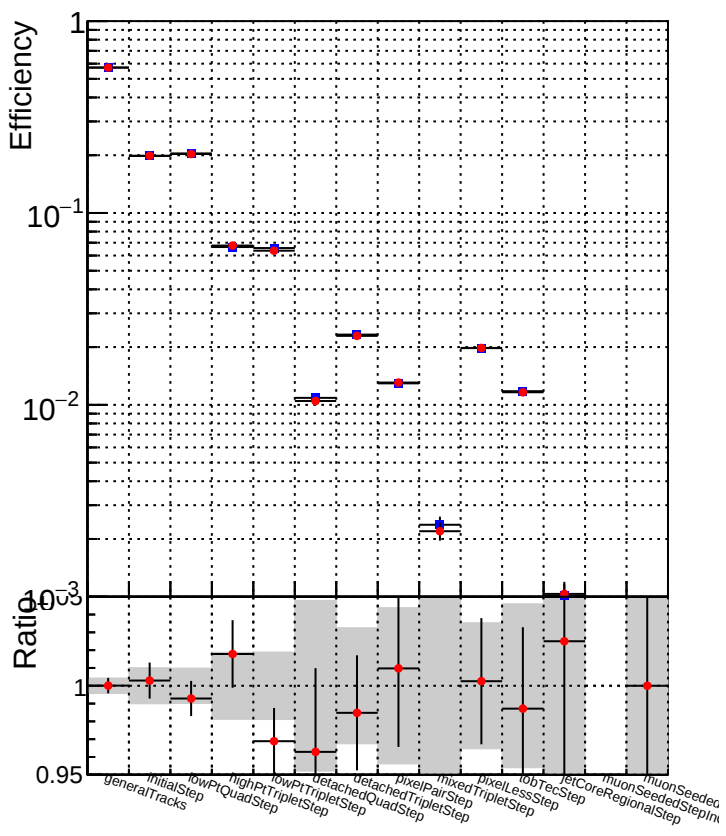
DQM_CKF_XiMinusNOPU_base DQM_CKF_XiMinusNOPU_retrainOldFiles125_v2_prelimWPM_epoch3
