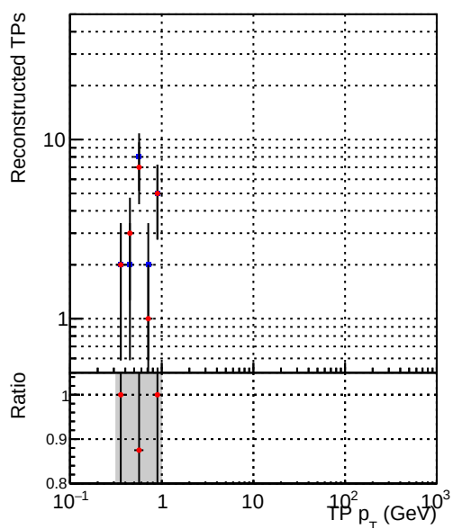
—•— DQM_CKF_XiMinusNOPU_base —•— DQM_CKF_XiMinusNOPU_retrainOldFiles125_v2_prelimWPM_epoch3
