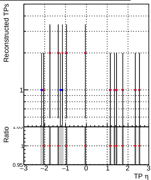
—•— DQM_CKF_XiMinusNOPU_base —•— DQM_CKF_XiMinusNOPU_retrainOldFiles125_v2_prelimWPM_epoch3
