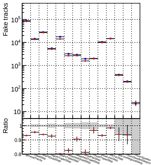
Number —●— DOM CKE XiMinusNOPU retrainOldFiles125 v2 prelimWPM epoch3
