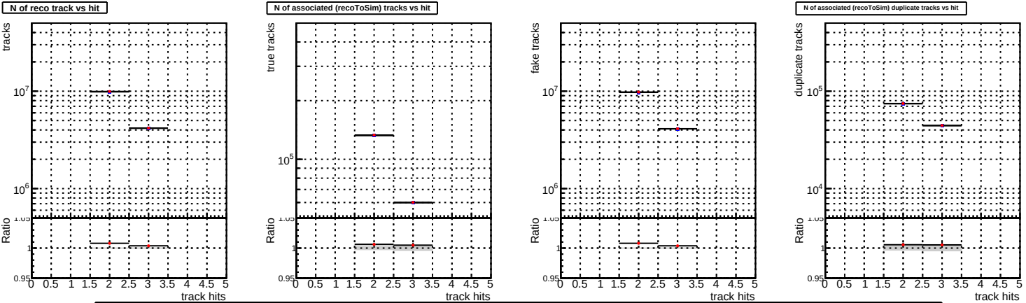
—•— DQM_CKF_XiMinusNOPU_base —•— DQM_CKF_XiMinusNOPU_retrainOldFiles125_v2_prelimWPM_epoch3
