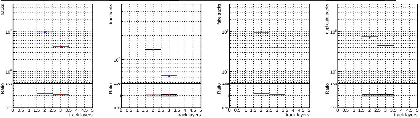
—•— DQM_CKF_XiMinusNOPU_base —•— DQM_CKF_XiMinusNOPU_retrainOldFiles125_v2_prelimWPM_epoch3
