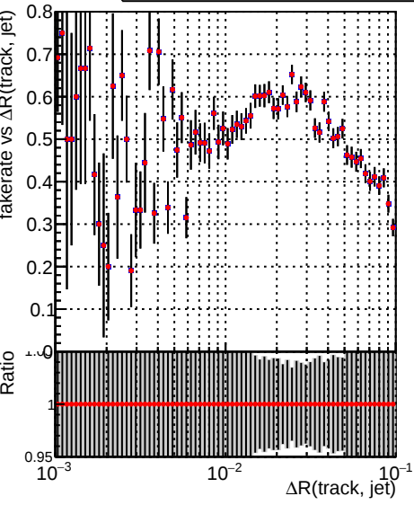
—•— DQM_CKF_XiMinusNOPU_base —•— DQM_CKF_XiMinusNOPU_retrainOldFiles125_v2_prelimWPM_epoch3
