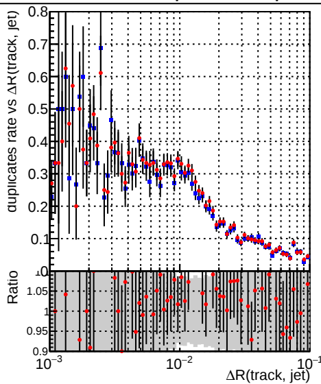
— DQM_CKF_XiMinusNOPU_base — DQM_CKF_XiMinusNOPU_retrainOldFiles125_v2_prelimWPM_epoch3
