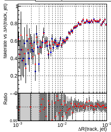
— DQM_CKF_XiMinusNOPU_base — DQM_CKF_XiMinusNOPU_retrainOldFiles125_v2_prelimWPM_epoch3
