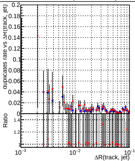
—•— DQM_CKF_XiMinusNOPU_base —•— DQM_CKF_XiMinusNOPU_retrainOldFiles125_v2_prelimWPM_epoch3
