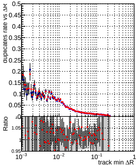
—•— DQM_CKF_XiMinusNOPU_base —•— DQM_CKF_XiMinusNOPU_retrainOldFiles125_v2_prelimWPM_epoch3
