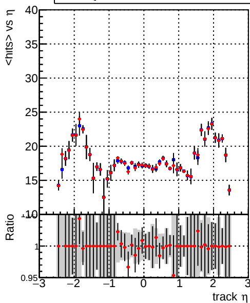
DQM_CKF_XiMinusNOPU_retrainOldFiles125_v2_prelimWPM_epoch3
