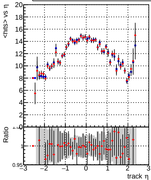
mean hits — DQM_CKF_XiMinusNOPU_base — DQM_CKF_XiMinusNOPU_retrainOldFiles125_v2_prelimWPM_epoch3
