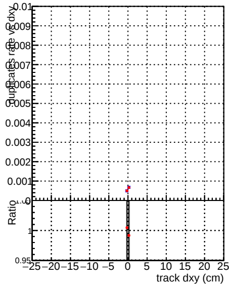
—●— DQM_CKF_XiMinusNOPU_base —●— DQM_CKF_XiMinusNOPU_retrainOldFiles125_v2_prelimWPM_epoch3
