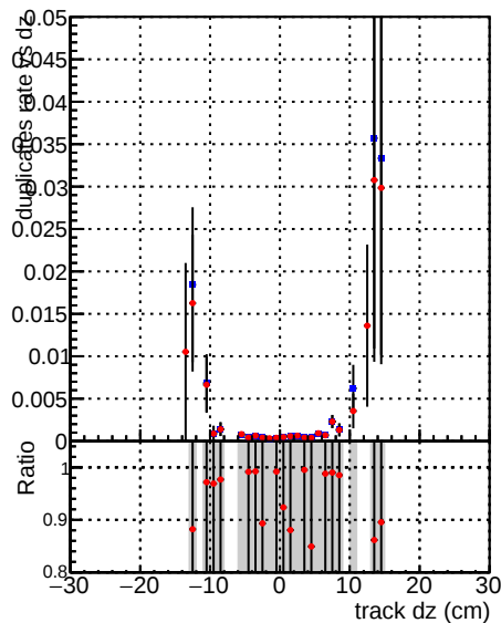
—●— DQM_CKF_XiMinusNOPU_base —●— DQM_CKF_XiMinusNOPU_retrainOldFiles125_v2_prelimWPM_epoch3
