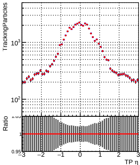
—•— DQM_CKF_XiMinusNOPU_base —•— DQM_CKF_XiMinusNOPU_retrainOldFiles125_v2_prelimWPM_epoch3
