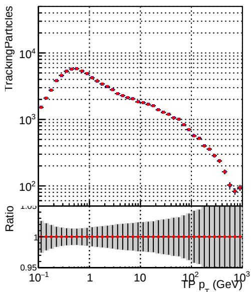
—•— DQM_CKF_XiMinusNOPU_base —•— DQM_CKF_XiMinusNOPU_retrainOldFiles125_v2_prelimWPM_epoch3
