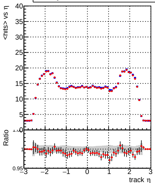
mean hits — DQM_CKF_XiMinusNOPU_base — DQM_CKF_XiMinusNOPU_retrainOldFiles125_v2_prelimWPM_epoch3
