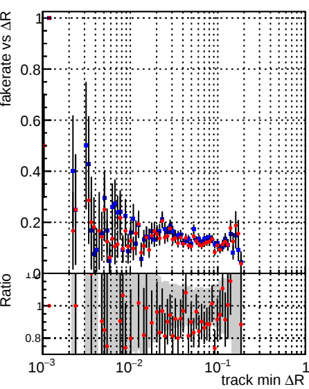
—•— DQM_CKF_XiMinusNOPU_base —•— DQM_CKF_XiMinusNOPU_retrainOldFiles125_v2_prelimWPM_epoch3
