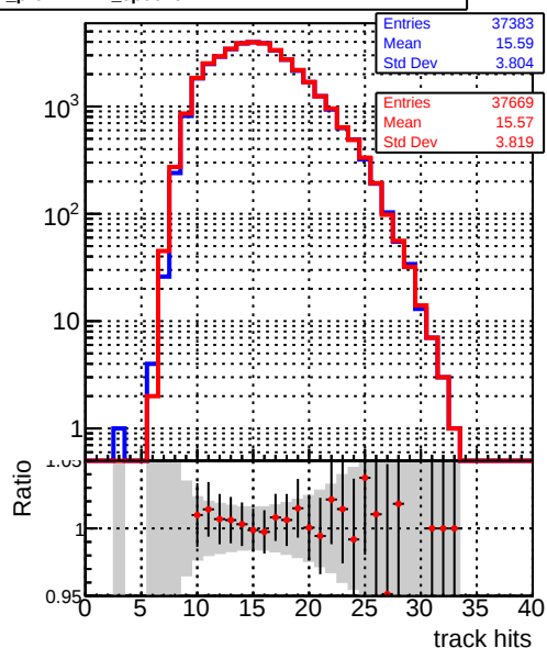
DQM_CKF_XiMinusNOPU_retrainOldFiles125_v2_prelimWPM_epoch3
