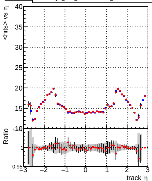
DQM_CKF_XiMinusNOPU_retrainOldFiles125_v2_prelimWPM_epoch3
