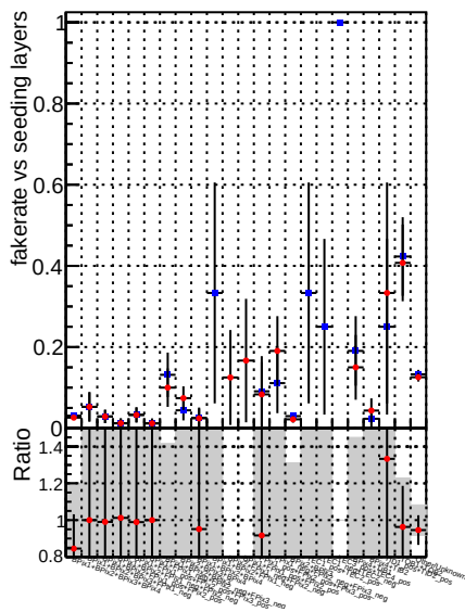
Fake rate vs. ◆ DQM CKF XiMinusNOPU_base ▲ DQM CKF XiMinusNOPU_retrainOldFiles125_v2_prelimWPM_epoch3
