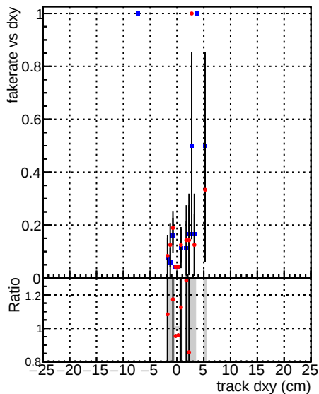
Fake rate vs d DQM CKF_XiMinusNOPU_base DQM CKF_XiMinusNOPU_retrainOldFiles125_v2_prelimWPM_epoch3
