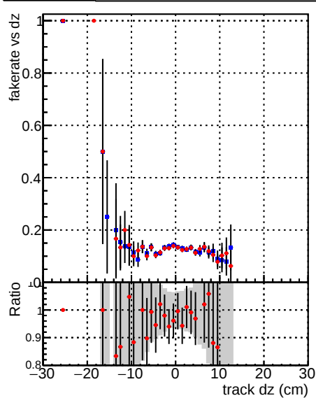
Fake rate vs dz DQM CKF XiMinusNOPU_base DQM CKF XiMinusNOPU_retrainOldFiles125_v2_prelimWPM_epoch3
