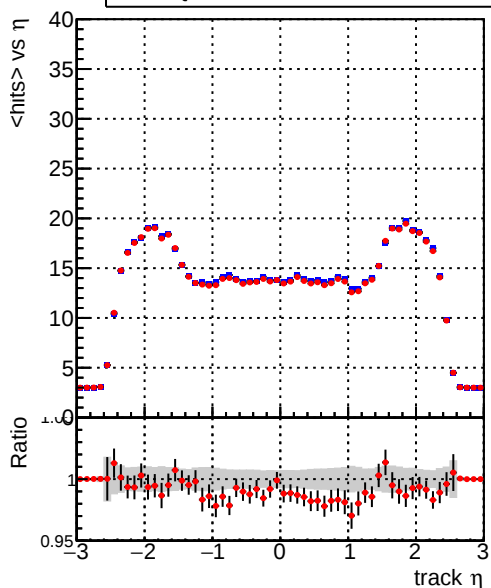
DQM_CKF_XiMinusNOPU_retrainOldFiles125_v2_prelimWPM_epoch3
