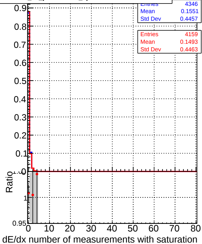
■ DQM_CKF_XiMinusNOPU_base ● DQM_CKF_XiMinusNOPU_retrainOldFiles125_v2_prelimWPM_epoch3
