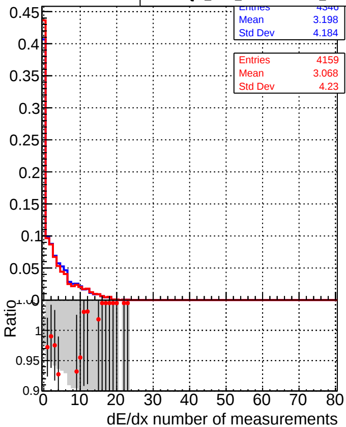
■ DQM_CKF_XiMinusNOPU_base ● DQM_CKF_XiMinusNOPU_retrainOldFiles125_v2_prelimWPM_epoch3
