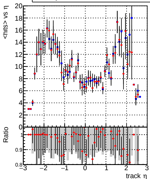
mean hits > \eta — DQM_CKF_XiMinusNOPU_base — DQM_CKF_XiMinusNOPU_retrainOldFiles125_v2_prelimWPM_epoch3
