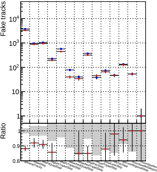
—●— DQM_CKF_XiMinusNOPU_retrainOldFiles125_v2_prelimWPM_epoch3
