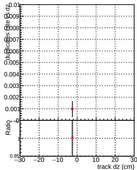
—●— DQM_CKF_XiMinusNOPU_base —●— DQM_CKF_XiMinusNOPU_retrainOldFiles125_v2_prelimWPM_epoch3
