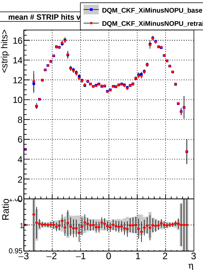
Legend: DQM_CKF_XiMinusNOPU_base DQM_CKF_XiMinusNOPU_retrainOldFiles125_v2_prelimWPM_epoch3
