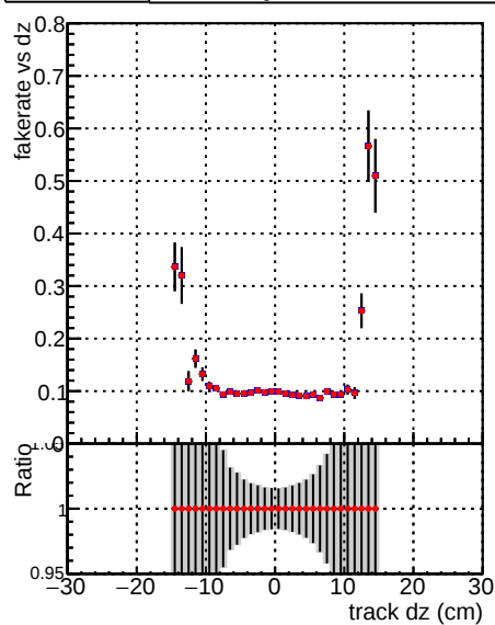
—•— DQM_CKF_XiMinusNOPU_base —•— DQM_CKF_XiMinusNOPU_retrainOldFiles125_v2_prelimWPM_epoch3
