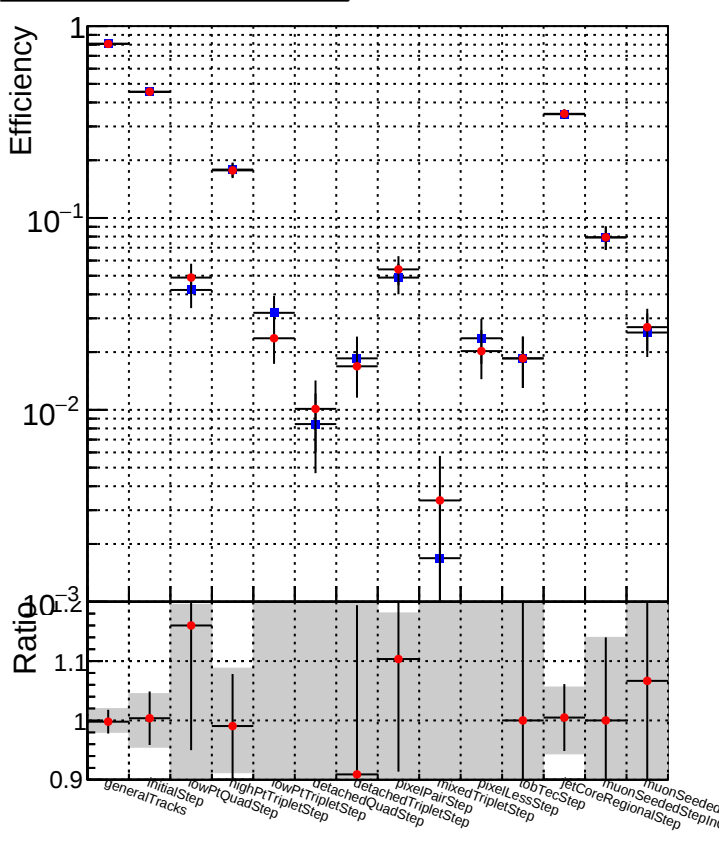
DQM_CKF_XiMinusNOPU_base DQM_CKF_XiMinusNOPU_retrainOldFiles125_v2_prelimWPM_epoch3
