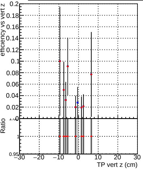
Efficiency vs TP vert z (cm) Legend: DQM_CKF_XiMinusNOPU_base DQM_CKF_XiMinusNOPU_retrainOldFiles125_v2_prelimWPM_epoch3
