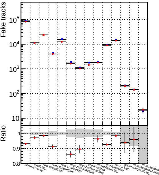
Numbe 1 DQM_CKF_XiMinusNOPU_retrainOldFiles125_v2_prelimWPM_epoch3
