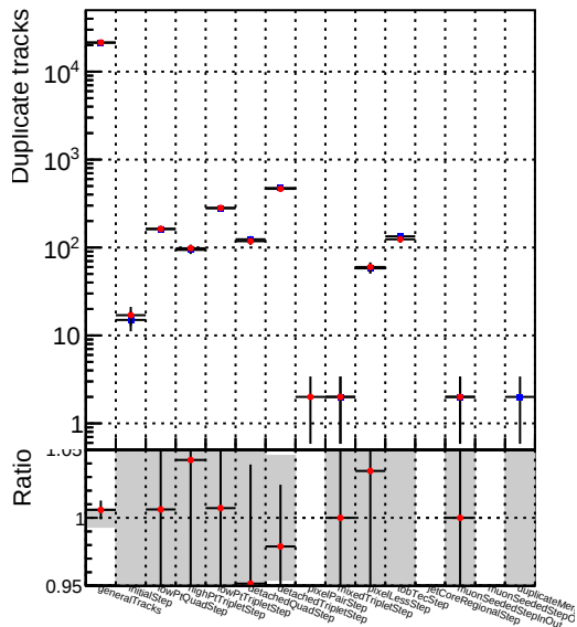
— DQM_CKF_XiMinusNOPU_v2_base Number —● DQM_CKF_XiMinusNOPU_retrainOldFiles125_v2_prelimWPM_epoch3
