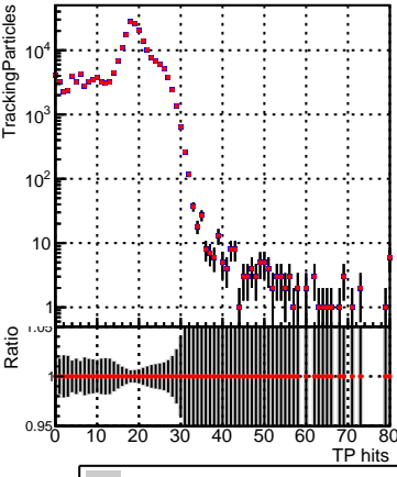
■ DQM_CKF_XiMinusNOPU_base ■ DQM_CKF_XiMinusNOPU_retrainOldFiles125_v2_prelimWPM_epoch3
