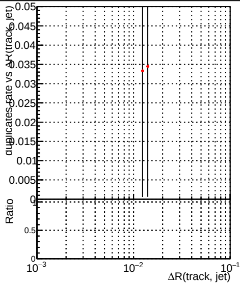
—●— DQM_CKF_XiMinusNOPU_base —●— DQM_CKF_XiMinusNOPU_retrainOldFiles125_v2_prelimWPM_epoch3
