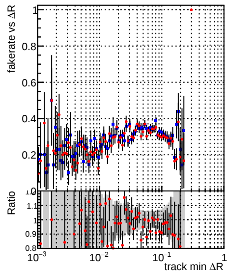
—●— DQM_CKF_XiMinusNOPU_base —●— DQM_CKF_XiMinusNOPU_retrainOldFiles125_v2_prelimWPM_epoch3
