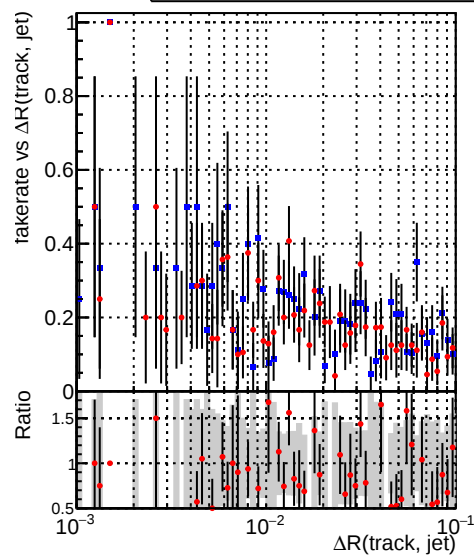
—●— DQM_CKF_XiMinusNOPU_base —●— DQM_CKF_XiMinusNOPU_retrainOldFiles125_v2_prelimWPM_epoch3
