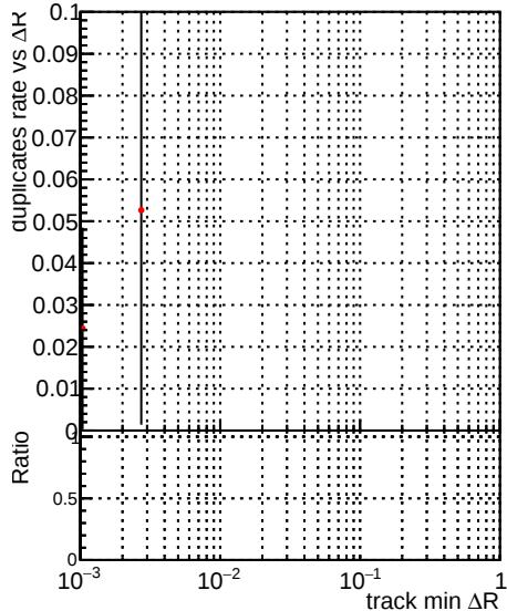
—●— DQM_CKF_XiMinusNOPU_base —●— DQM_CKF_XiMinusNOPU_retrainOldFiles125_v2_prelimWPM_epoch3
