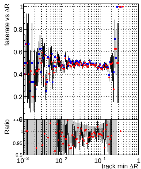
—●— DQM_CKF_XiMinusNOPU_base —●— DQM_CKF_XiMinusNOPU_retrainOldFiles125_v2_prelimWPM_epoch3
