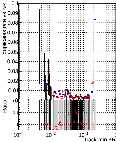
—●— DQM_CKF_XiMinusNOPU_base —●— DQM_CKF_XiMinusNOPU_retrainOldFiles125_v2_prelimWPM_epoch3
