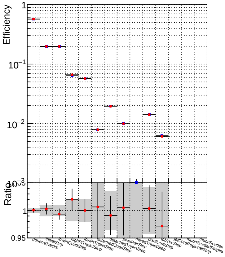
DQM_CKF_XiMinusNOPU_base DQM_CKF_XiMinusNOPU_retrainOldFiles125_v2_prelimWPM_epoch2
