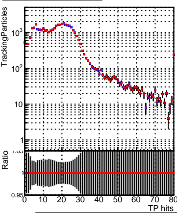
■ DQM_CKF_XiMinusNOPU_base ■ DQM_CKF_XiMinusNOPU_retrainOldFiles125_v2_prelimWPM_epoch2
