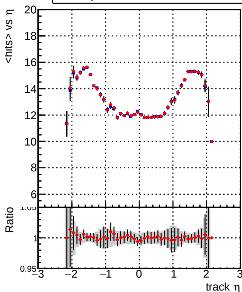
mean hits — DQM_CKF_XiMinusNOPU_base — DQM_CKF_XiMinusNOPU_retrainOldFiles125_v2_prelimWPM_epoch2
