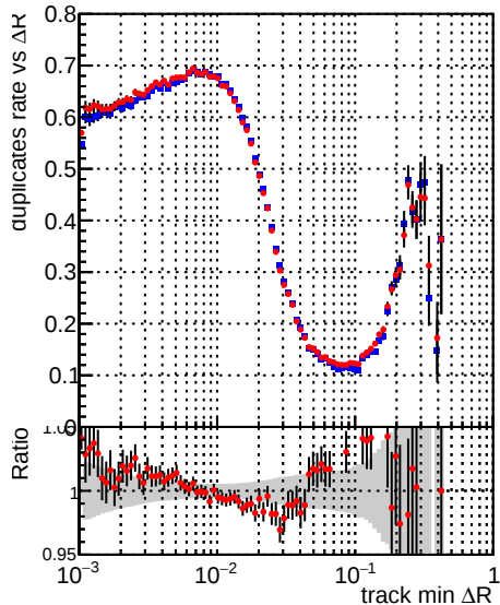
■ DQM_CKF_XiMinusNOPU_base ● DQM_CKF_XiMinusNOPU_retrainOldFiles125_v2_prelimWPM_epoch2
