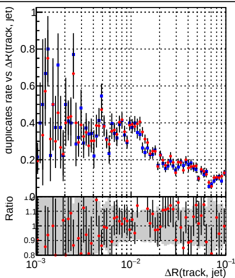
■ DQM_CKF_XiMinusNOPU_base ● DQM_CKF_XiMinusNOPU_retrainOldFiles125_v2_prelimWPM_epoch2
