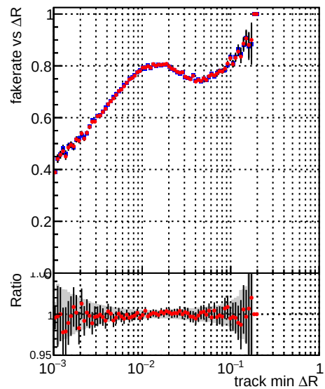
—•— DQM_CKF_XiMinusNOPU_base —•— DQM_CKF_XiMinusNOPU_retrainOldFiles125_v2_prelimWPM_epoch2
